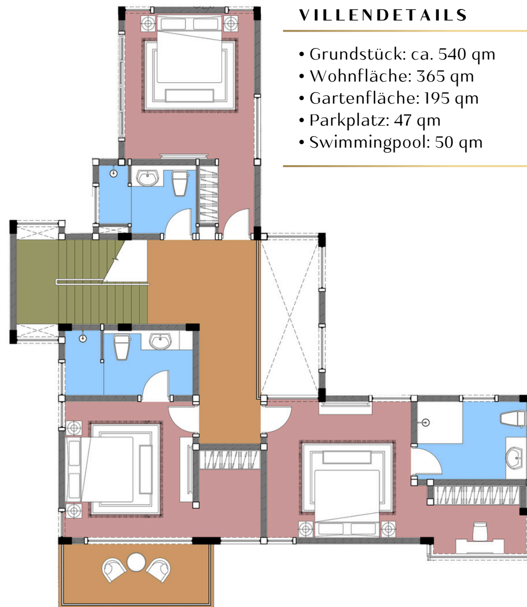
GRUNDRISS OBERGESCHOSS
